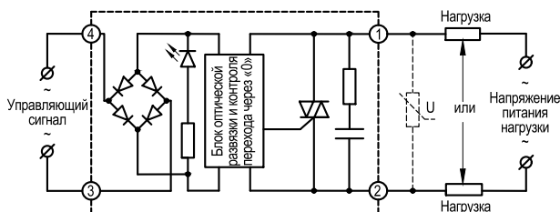
Рисунок 10 – схема подключения ТТР серии HD-хх44.ZA2 (модификации с симисторным выходом)
