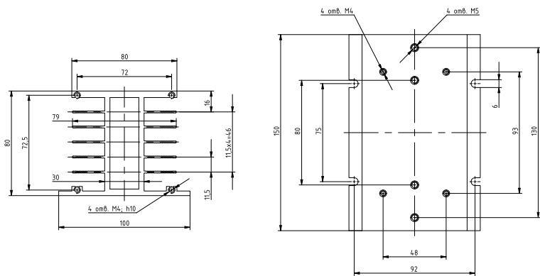
Рисунок 54 – габаритные и установочные размеры радиатора PTP036
