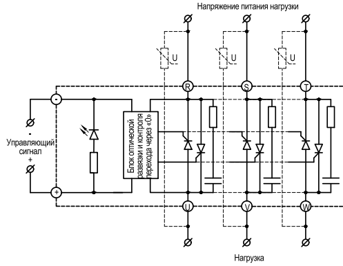
Рисунок 32 – схема подключения ТТР серии HT-xx44.ZD3 (≥100 А)
