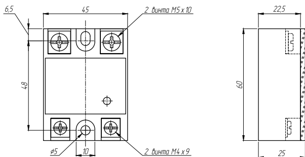
Рисунок 15 – габаритные и установочные размеры ТТП серии HD-xx22.10U
