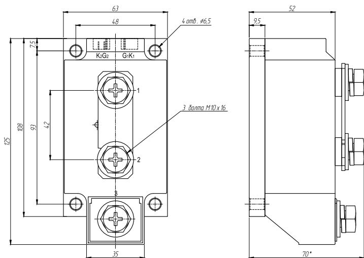
Рисунок 25 – габаритные и установочные размеры ТТР серии GaDH-800120.ZD3
