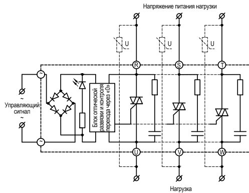
Рисунок 33 – схема подключения ТТР серии HT-xx44.ZA2 (≤40 А)
