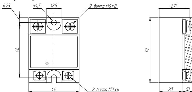
Рисунок 8 – габаритные и установочные размеры ТТП серий HD-xx44.ZD3 / ZA2
