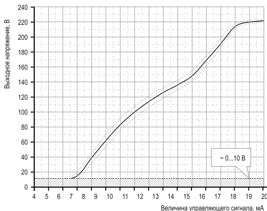
Рисунок 45 – зависимость выходного напряжения от входного сигнала ТТП серии HD-xx25.LA
