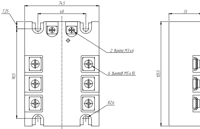
Рисунок 29 – габаритные и установочные размеры ТТР серий НТ-хх44.ZD3 / ZA2
