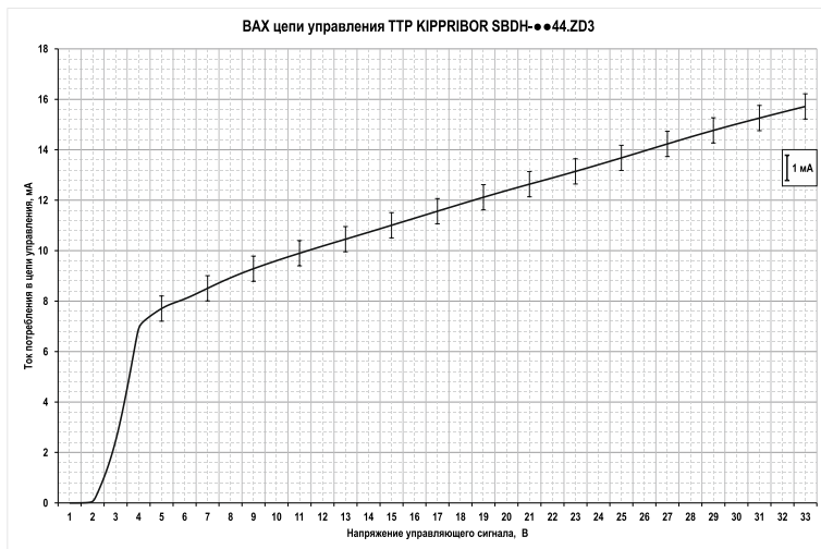
Рисунок 39 – ВАХ входной цепи ТТР серии SBDH-xx44.ZD3
