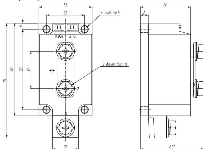
Рисунок 24 – габаритные и установочные размеры ТТР серий GaDH-500120.ZD3, GaDH-600120.ZD3
