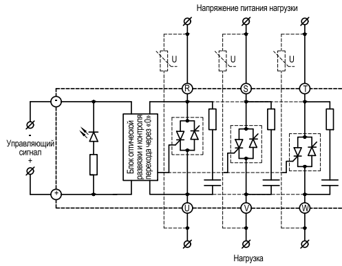
Рисунок 31 – схема подключения ТТР серии HT-xx44.ZD3 (60 и 80 А)
