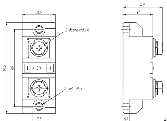
Рисунок 22 – габаритные и установочные размеры ТТП серии BDH-xx44.ZD3
