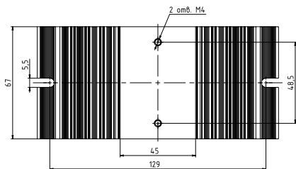
Рисунок 50 – габаритные и установочные размеры радиатора РТР061.1
