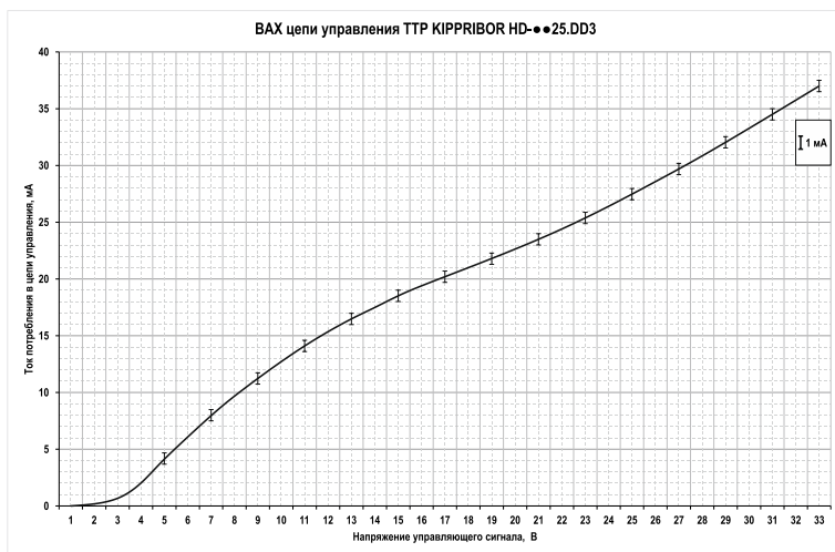
Рисунок 37 – ВАХ входной цепи ТТР серии HD-xx25.DD3
