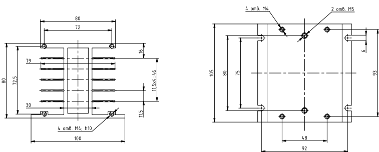
Рисунок 53 – габаритные и установочные размеры радиатора PTP034
