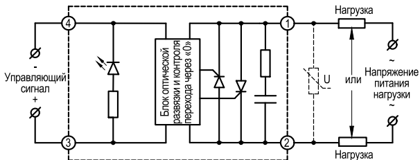
Рисунок 20 – схема подключения ТТР серии HDH-xx44.ZD3
