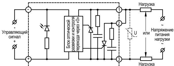
Рисунок 28 – схема подключения ТТР серий GaDH / GwDH-xxx120.ZD3
