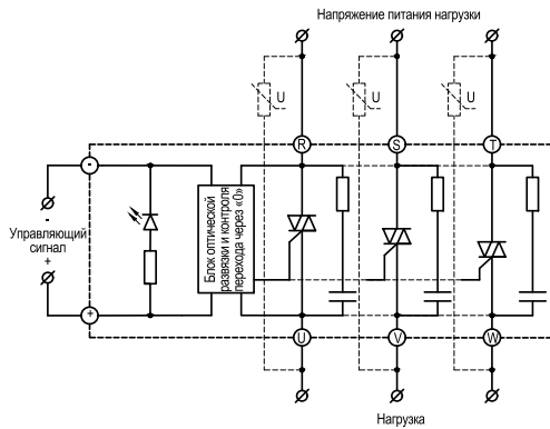
Рисунок 30 – схема подключения ТТР серии НТ-хх44.ZD3 ( \leq 40 А)
