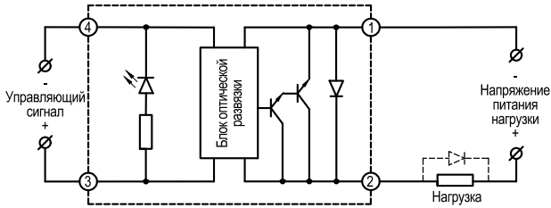
Рисунок 13 – схема подключения ТТР серии HD-xx25.DD3
