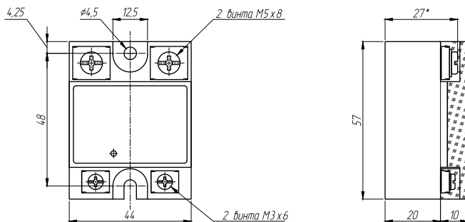
Рисунок 14 – габаритные и установочные размеры ТТР серий HD-xx44.VA, HD-xx25.LA
