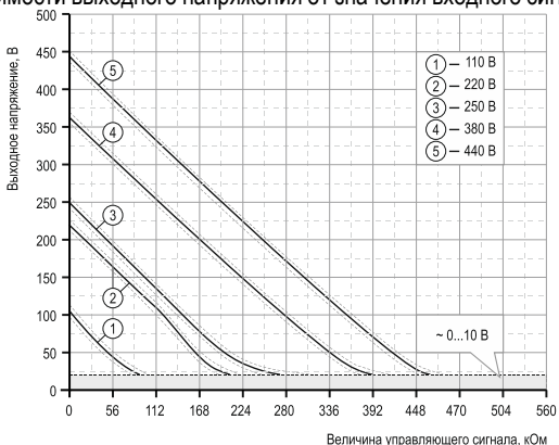
Рисунок 43 – зависимость выходного напряжения от входного сигнала ТТР серии HD-xx44.VA
