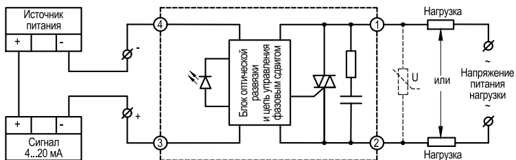
Рисунок 17 – схема подключения ТТП серий HD-xx25.LA
