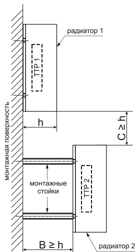
Рисунок 60 – схема размещения ТТР при монтаже друг над другом
