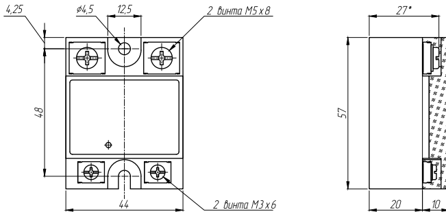
Рисунок 19 – габаритные и установочные размеры ТТР серии HDH-xx44.ZD3
