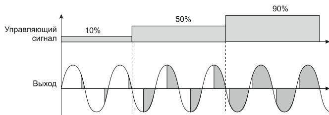
Рисунок 47 – диаграмма срабатывания ТТР с фазовым управлением
