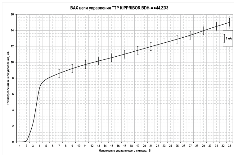
Рисунок 40 – ВАХ входной цепи ТТР серии BDH-xx44.ZD3
