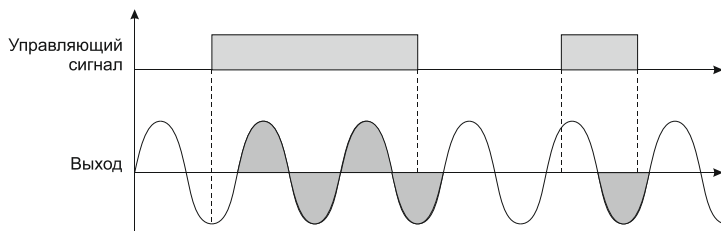
Рисунок 46 – диаграмма срабатывания ТТР с контролем перехода через ноль
