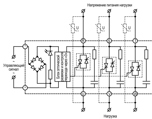
Рисунок 34 – схема подключения ТР серии НТ-хх44.ZA2 ( \geq 60 A)
