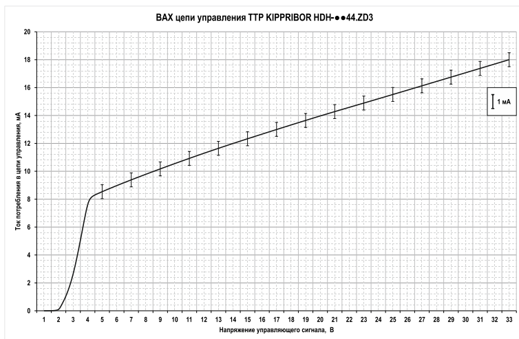
Рисунок 38 – ВАХ входной цепи ТТР серии HDH-xx44.ZD3
