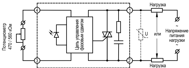
Рисунок 16 – схема подключения ТТП серии HD-xx44.VA
