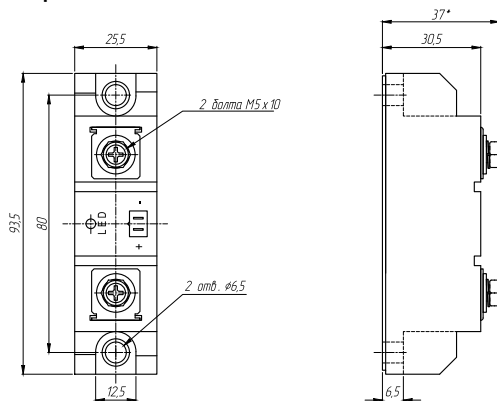
Рисунок 21 – габаритные и установочные размеры ТТР серии SBDH-xx44.ZD3
