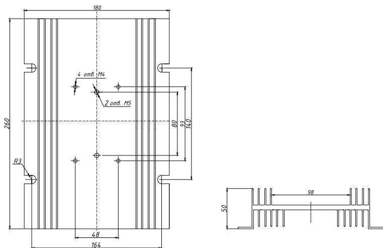
Рисунок 55 – габаритные и установочные размеры радиатора PTP037
