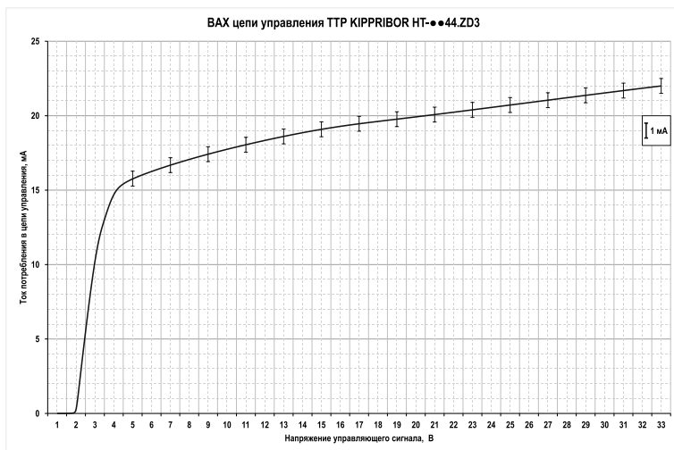
Рисунок 42 – ВАХ входной цепи ТТР серии HT-xx44.ZD3
