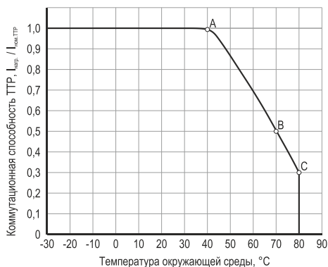
Рисунок 61 – зависимость тока реле от температуры окружающей среды (основания ТТР).
