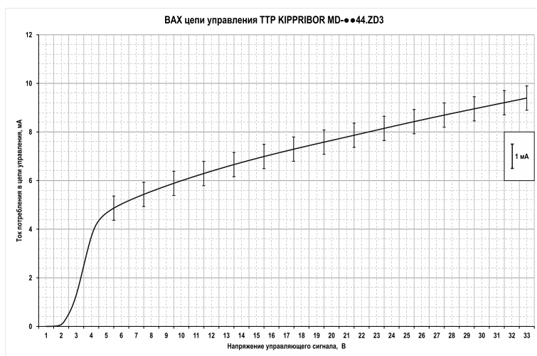
Рисунок 35 – ВАХ входной цепи ТТР серии MD-xx44.ZD3
