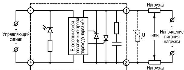
Рисунок 23 – схема подключения ТТП серий BDH / SBDH-xx44.ZD3
