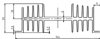
Рисунок 50 – габаритные и установочные размеры радиатора РТР061.1
