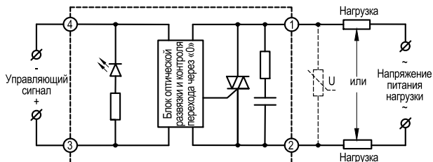
Рисунок 9 – схема подключения ТТП серий HD-xx44.ZD3
