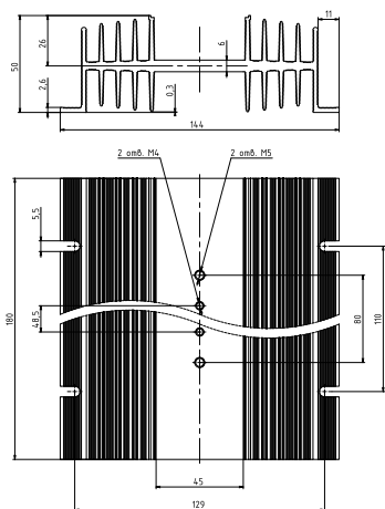
Рисунок 52 – габаритные и установочные размеры радиатора PTP063.1
