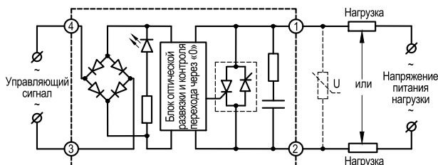
Рисунок 11 – схема подключения ТТР серии HD-хх44.ZA2 (модификации с тиристорным выходом)
