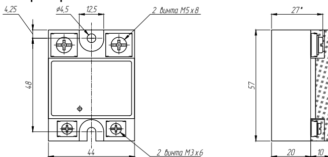
Рисунок 12 – габаритные и установочные размеры ТТП серии HD-xx25.DD3
