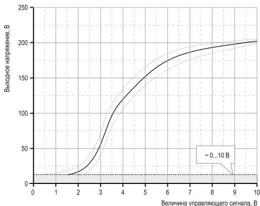
Рисунок 44 – зависимость выходного напряжения от входного сигнала ТТР серии HD-xx22.10U
