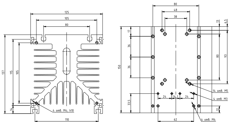
Рисунок 56 – габаритные и установочные размеры радиатора РТР038
