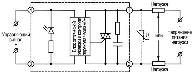
Рисунок 7 – схема подключения ТТР серии MD-xx44.ZD3
