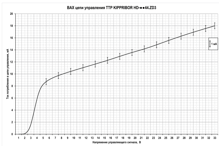
Рисунок 36 – ВАХ входной цепи ТТР серии HD-xx44.ZD3
