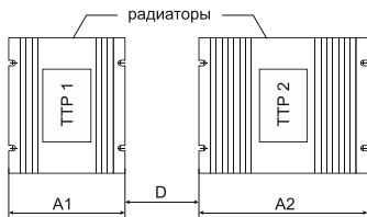
Рисунок 59 – схема размещения ТТР при монтаже в одном ряду
