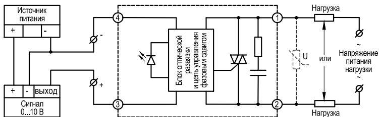
Рисунок 18 – схема подключения ТТР серии HD-xx22.10U
