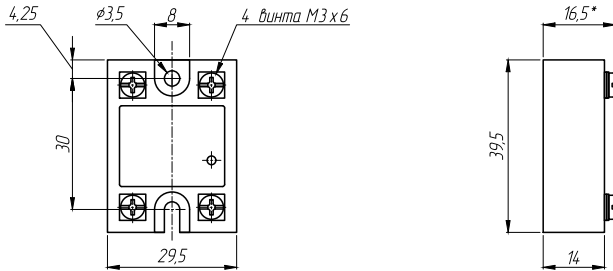
Рисунок 6 – габаритные и установочные размеры ТТР серии MD-xx44.ZD3
