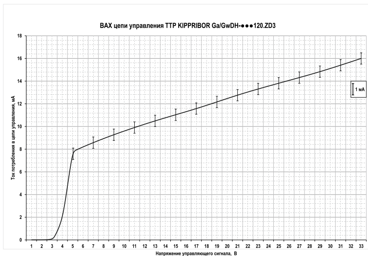
Рисунок 41 – ВАХ входной цепи ТТР серии (Ga)GwDH-xx120.ZD3
