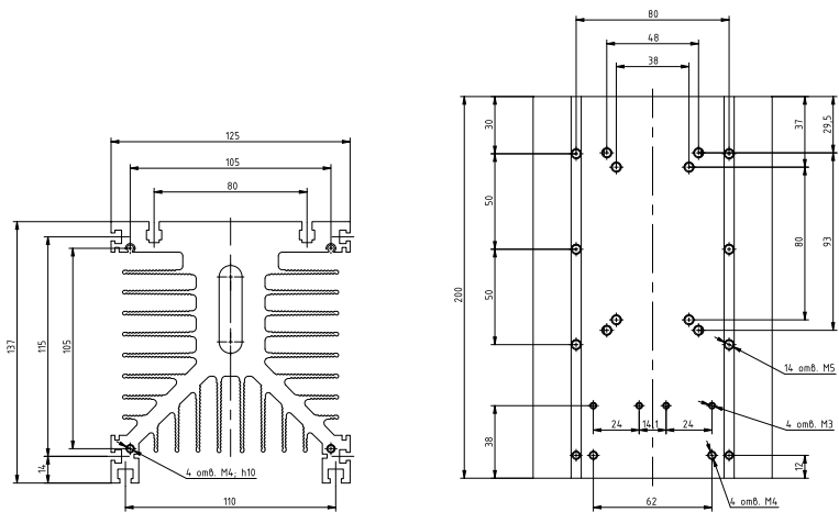
Рисунок 57 – габаритные и установочные размеры радиатора РТР039
