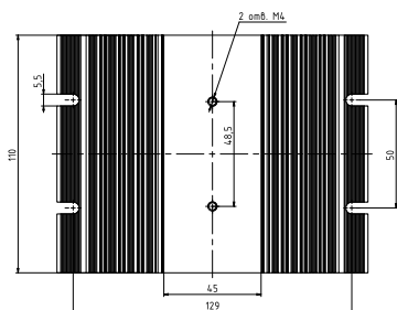
Рисунок 51 – габаритные и установочные размеры радиатора РТР062.1
