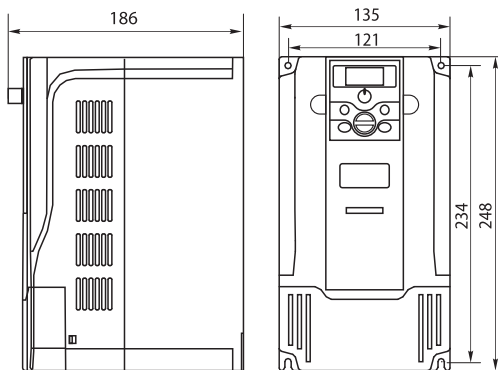
Габарит корпуса 4
