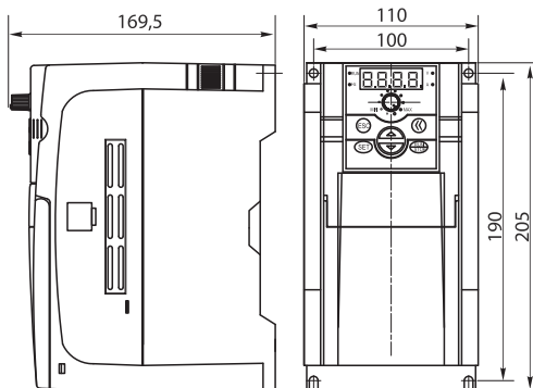
Габарит корпуса 3
